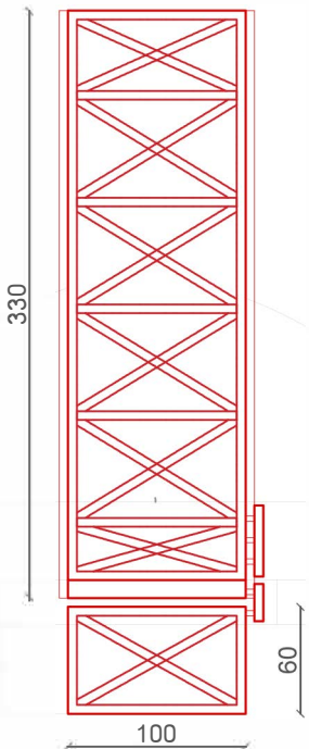
PLANSTRUKTURE
