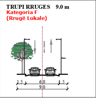
PRERJA 6-6
