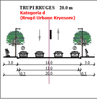
PRERJA 1-1
