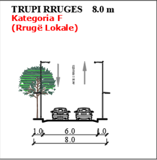
PRERJA 3-3
