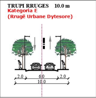
PRERJA 2-2
