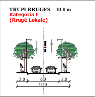
PRERJA 5-5
