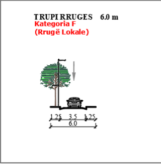
PRERJA 4-4
