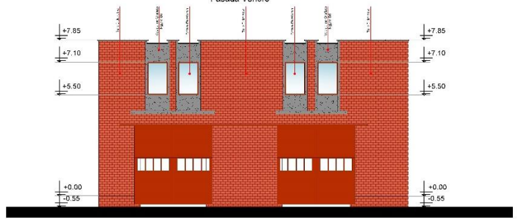
Fasada Veriore
