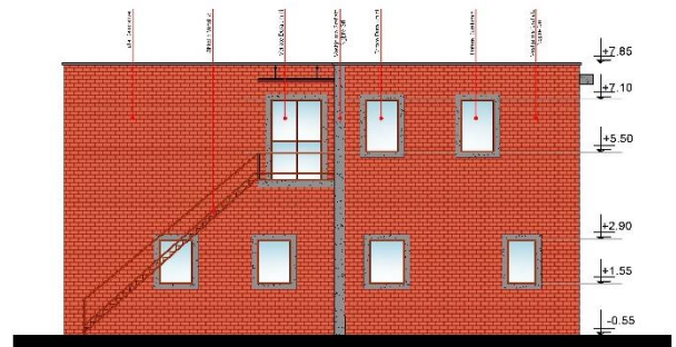
Fasada Jugore
