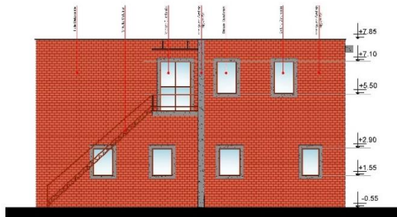
Fasada Jugore
